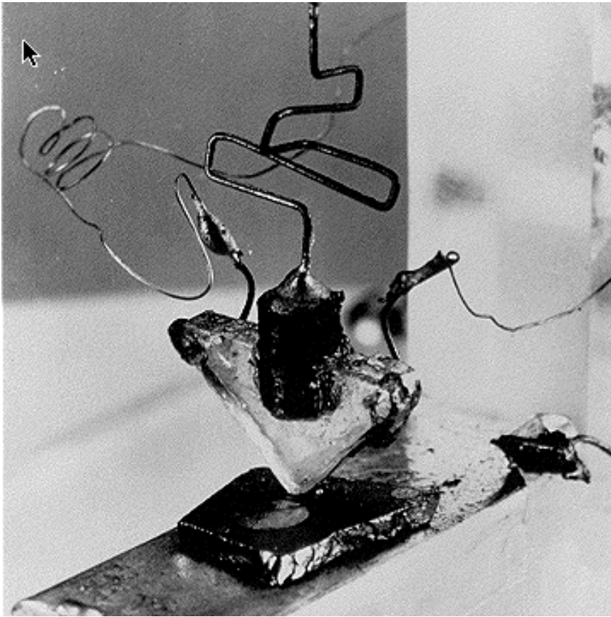
1º transistor (Bell Labs, EUA, 1947)
