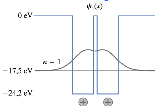
Orbital Ligante
