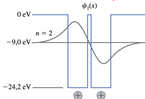
Orbital Anti-Ligante
