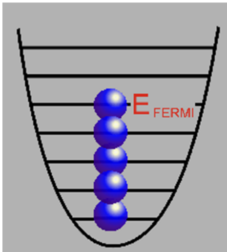
Férmions
